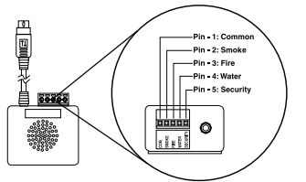
Figure 3 : Connexions Contact Closure [fermeture à contact] d'EnviroSense
